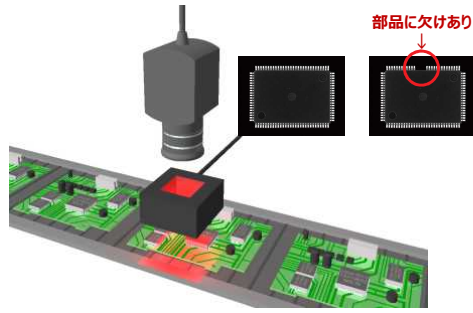
プリント基板の実装部品欠陥検査
